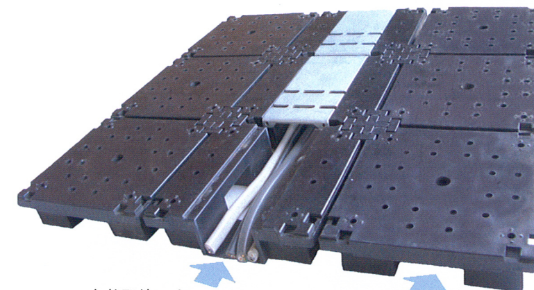
有効配線スペース 40x21mm
